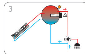
Sistema de termosifón (página 11)
