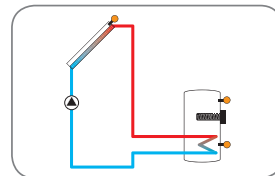
Sistema de energía solar estándar con 1 acumulador y calentamiento auxiliar eléctrico (página 13)
